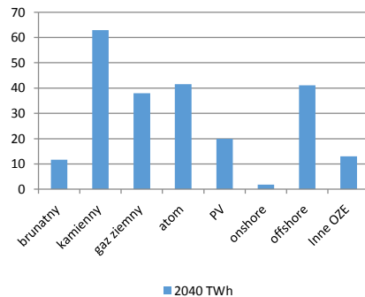
Produkcja energii w 2040 roku wg. PEP 2040 [TWh]
